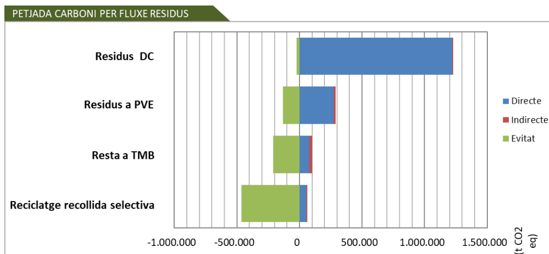
Figura 4. Petjada de carboni del tractament de residus municipals de Catalunya (2016) per flux de residus
