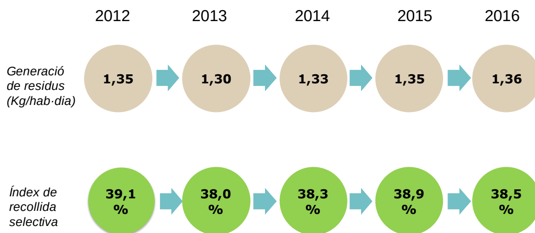
Figura A. Generació de residus per càpita i índex de recollida selectiva (2012-2016)
