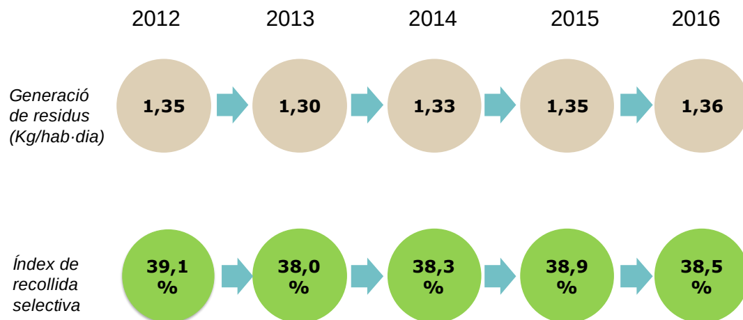
Figura 8. Generació de residus i índex de recollida selectiva (2012-2016)
