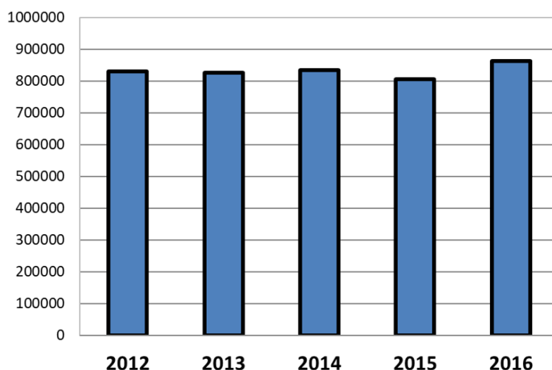
Figura 12. Evolució de la petjada de carboni de Catalunya (2012-2016). Dades expressades en tones de CO 2 eq
