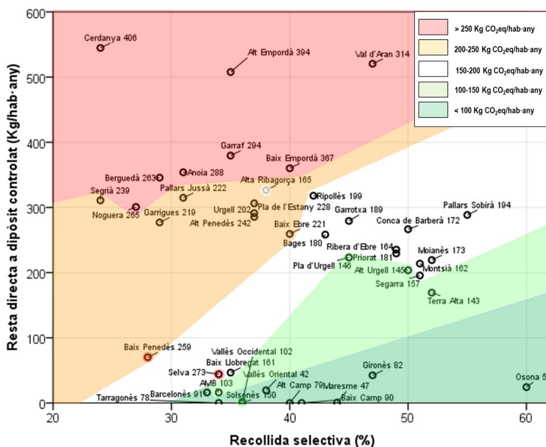
Figura C. Diagrama de dispersió de la recollida selectiva i de la resta enviada a dipòsit controlat per habitant, per comarca (2016). El número que acompanya el nom de la comarca correspon a la petjada de carboni de la gestió de residus municipals (Kg CO 2 eq/hab·any).
