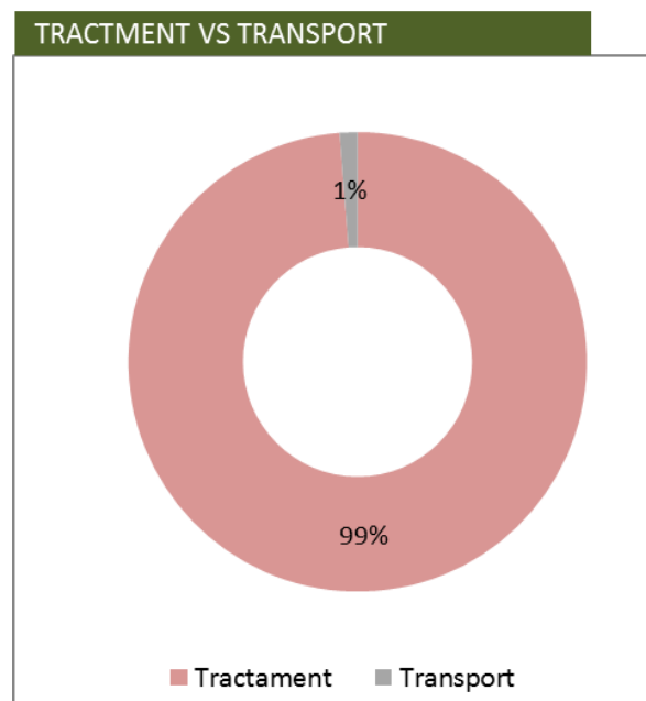
Figura 6. Contribució del transport al total d'impactes generats per la gestió dels residus municipals a Catalunya (2016)
