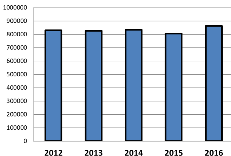
Figura B. Evolució de la petjada de carboni total en el període 2012-2016.
