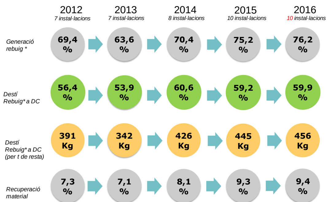
Figura 10. Evolució de les plantes de TMB de Catalunya (2012-2016). Les dades de rebuig, inclouen també el bioestabilitzat amb destí dipòsit controlat.
