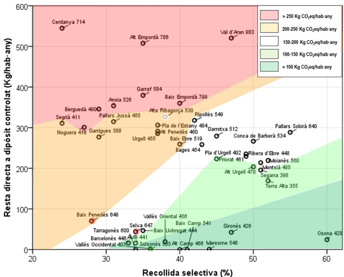
Figura 18. Diagrama de dispersió de la recollida selectiva i de la resta enviada a dipòsit controlat per habitant, per comarca (2016). El número que acompanya el nom de la comarca correspon a la generació de residus per habitant (Kg/hab·any). La llegenda de colors indica el rang en què es situa la petjada de carboni per habitant (Kg CO 2 eq/hab·any)
