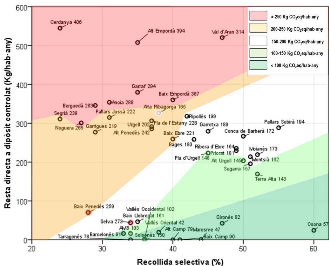
Figura 17. Diagrama de dispersió de la recollida selectiva i de la resta enviada a dipòsit controlat per habitant, per comarca (2016). El número que acompanya el nom de la comarca correspon a la petjada de carboni de la gestió de residus municipals (Kg CO 2 eq/hab·any)
