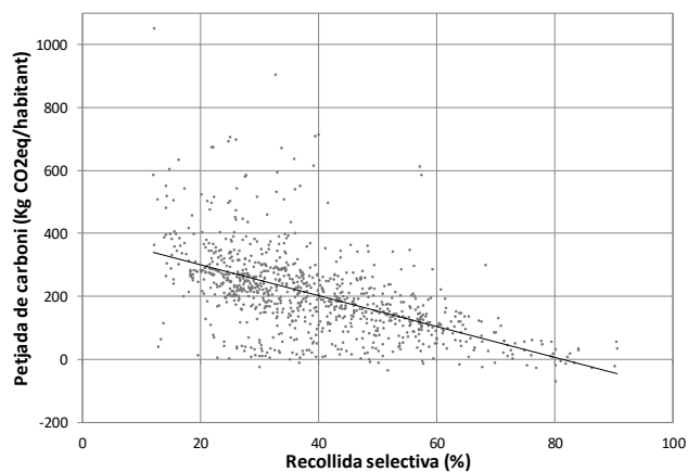
Figura 15. Models de regressió lineal de la petjada de carboni per habitant i la resta a dipòsit controlat, generació de residus i recollida selectiva, respectivament (2016).
