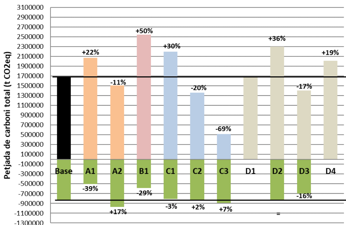
Figura 7. Emissions generades i evitades de la gestió dels residus municipals a Catalunya (2016): escenari base vs escenaris alternatius
