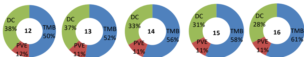
Figura 9. Destí de la fracció Resta a Catalunya (2012-2016). Nota: DC: Dipòsit Controlat, PVE: Planta Valorització Energètica; TMB: Tractament Mecànic-Biològic
