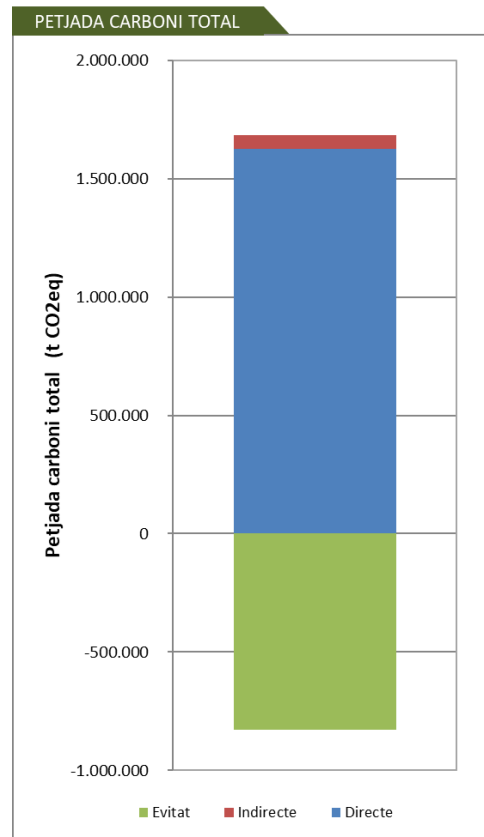
Figura 3. Petjada de carboni de Catalunya (2016): impactes directes, indirectes i evitats
