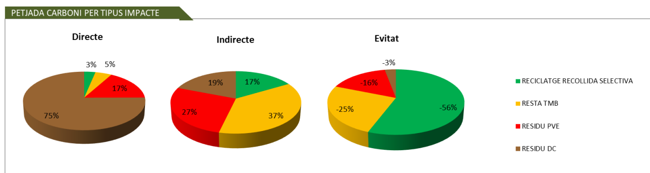
Figura 5. Petjada de carboni del tractament dels residus municipals a Catalunya (2016), per tipus d'impacte
