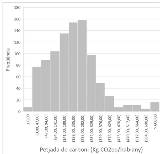
Figura 14. Histograma de la petjada de carboni de la gestió dels residus municipals dels municipis catalans (2016)
